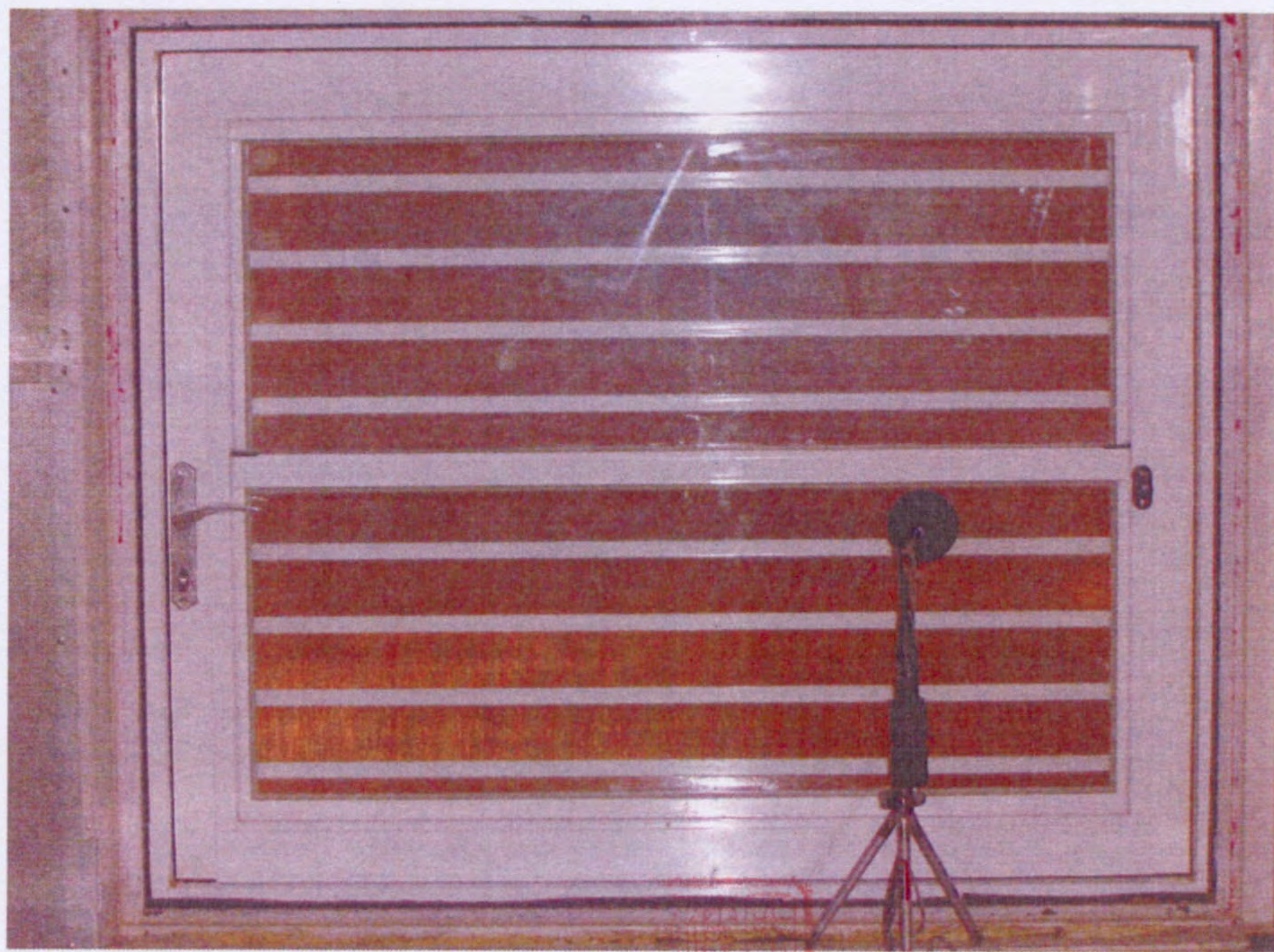
圖 1 試樣佈置圖 (無響室)
